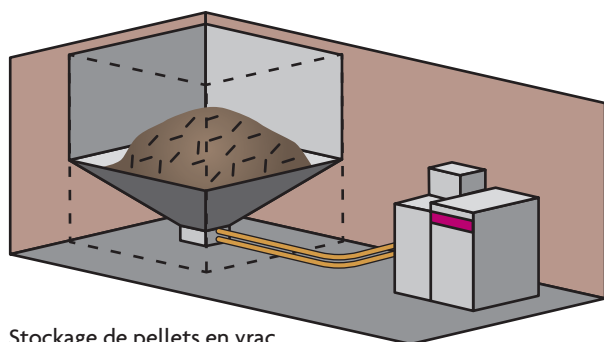
Stockage de pellets en vrac
